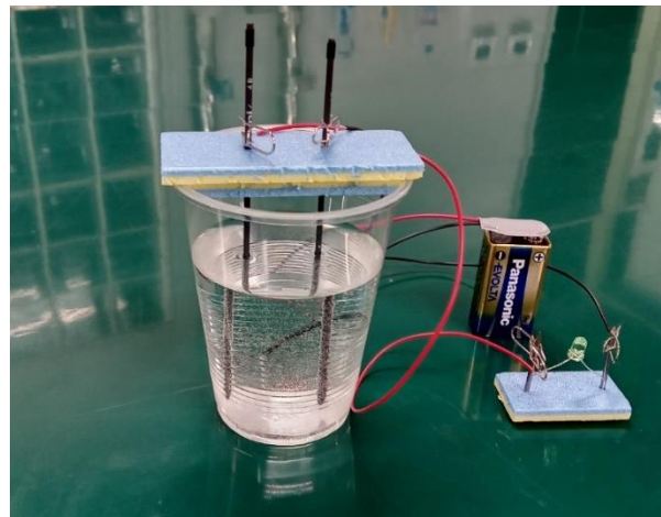
水素発生装置
